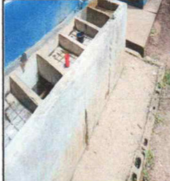
FOTO 2. REPARACION DE MURO CON BLOCK DE 50KG/CM2 14X19X39 + MALLA GALVANIZADA
