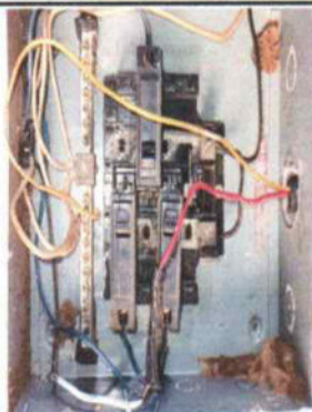
FOTO 9. REPARACION CABLEADO ELECTRICO CAL. 12AWG AULAS
