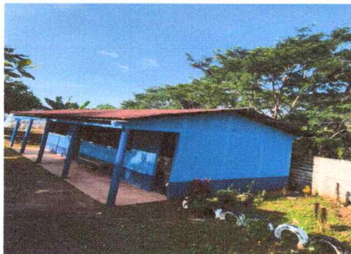
Sustitución de lámina por lámina troquelada calibre 26 Aluzinc
