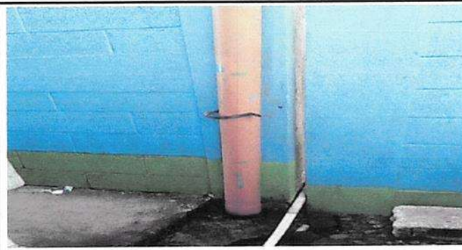
Foto 8: Sustrucción de bajadas de agua pluvial de metal por tubo pvc 3"
