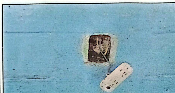
Foto 9: SUSTITUCIÓN DE TOMACORRIENTES DOBLES POLARIZADO 15A EAGLE. TOTAL 15 TOMACORRIENTES
