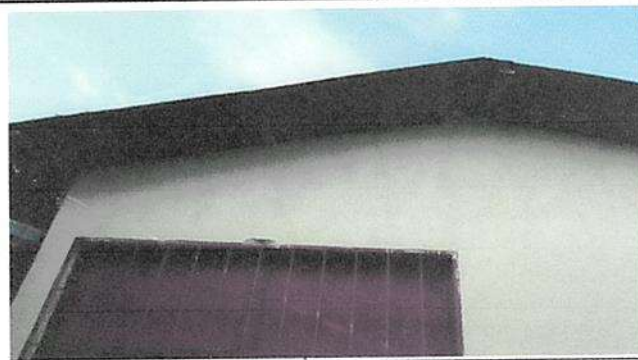
SUSTITUCION DE CUBIERTA DE LAMINA ACANALADA POR LAMINA TROQUELADA CALIBRE 26 ALUZINC
