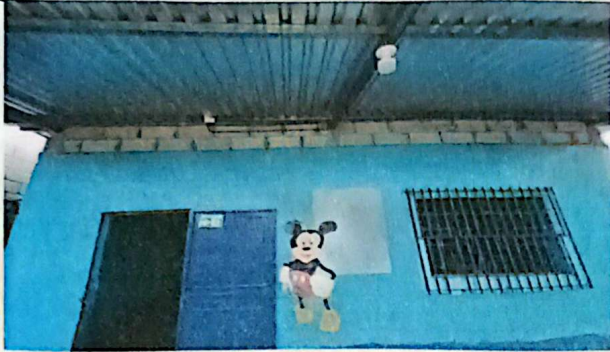
FOTOGRAFIA 7. INSTALACION DE CABLEADO ELECTRICO CALIBRE 8 AWG VIAKON, 14 AULAS, PASILLOS Y CORREDORES, TOTAL 315 METROS LINEALES
