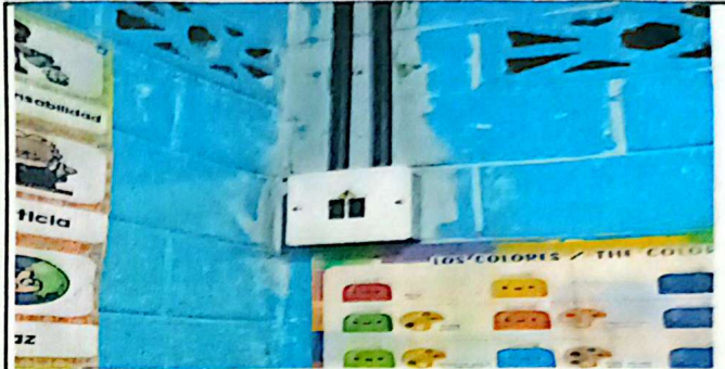
FOTOGRAFIA 8. INSTALACION DE CAJA DE DISTRIBUCION PLASTICA 4 MODULOS Y FLIPON AUTOMATICO NXB-63 2P 20A CHINT, 14 AULAS Y CENTRAL. TOTAL 15 CAJAS
