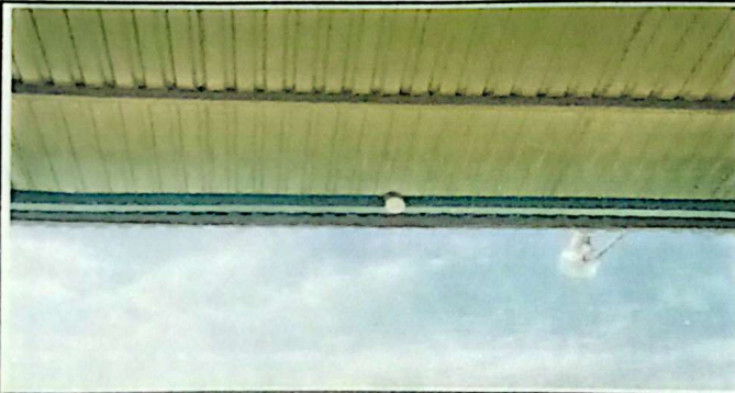
FOTOGRAFIA 1. SUSTITUCIÓN DE BOMBILLO LED GLOBO 30W 2400 LÚMENES. 14 AULAS Y CANCHA DEPORTIVA. TOTAL 75 BOMBILLOS
