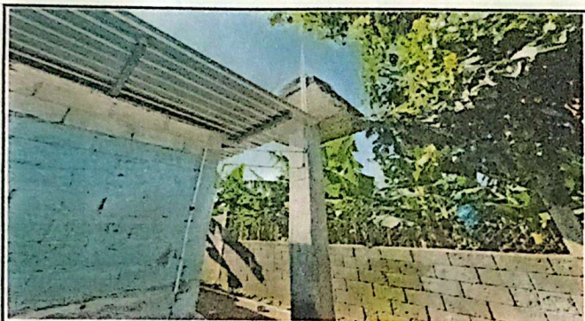
FOTOGRAFIA 9. INSTALACION DE SISTEMA DE AGUA POTABLE CON ELECTROVALVULA DE LLENADO. TOTAL 2 SISTEMAS
