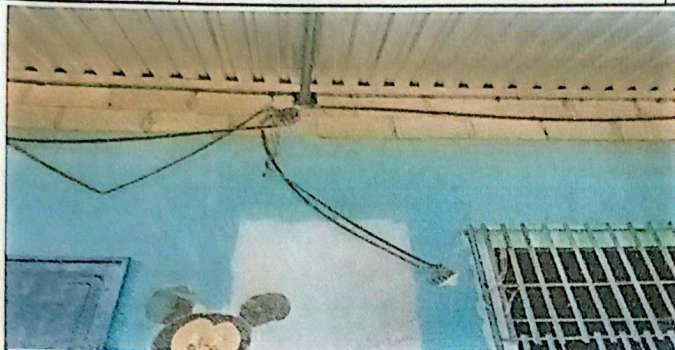
FOTOGRAFIA 7. INSTALACION DE CABLEADO ELECTRICO CALIBRE 8 AWG VIAKON, 14 AULAS, PASILLOS Y CORREDORES. TOTAL 315 METROS LINEALES
