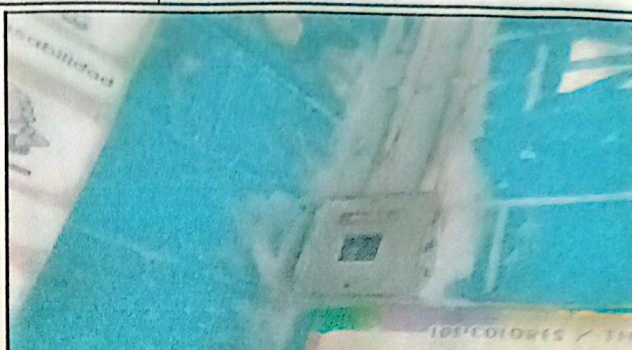
FOTOGRAFIA 8. INSTALACION DE CAJA DE DISTRIBUCION PLASTICA 4 MODULOS Y FLIPON AUTOMATICO NXB-63 2P 20A CHINT, 14 AULAS Y CENTRAL. TOTAL 15 CAJAS
