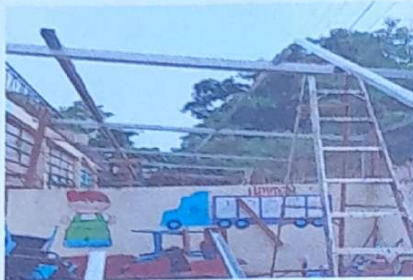
Foto 3: Sustitución de estructura de madera a estructura metálica con costanera galvanizada.
