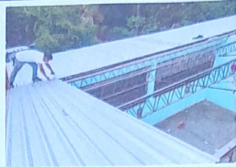
Foto 2: Reparación de estructura portante con tubo de 1" X 1 1/2" + colocación de lamina troquelada calibre 26 modulo 2
