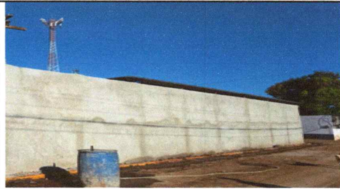
Foto 2: Reparación de Muro con Block 50Kg7cm2 14x19x39 cm
