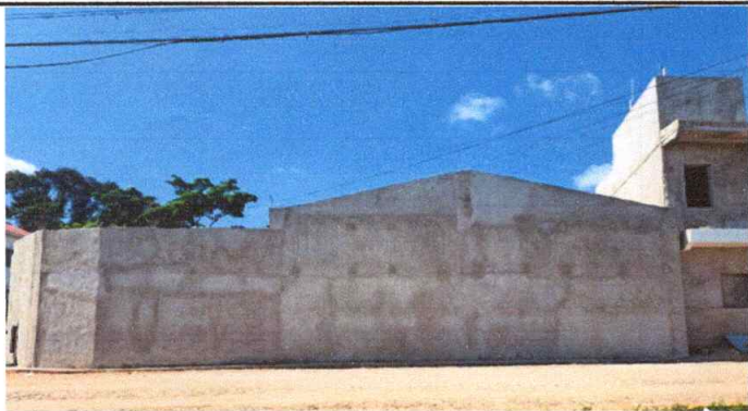
Foto 1: Reparación de muro con Columnas 0.20x0.20x4.0m 4 Hierro 1/2 y estribos
