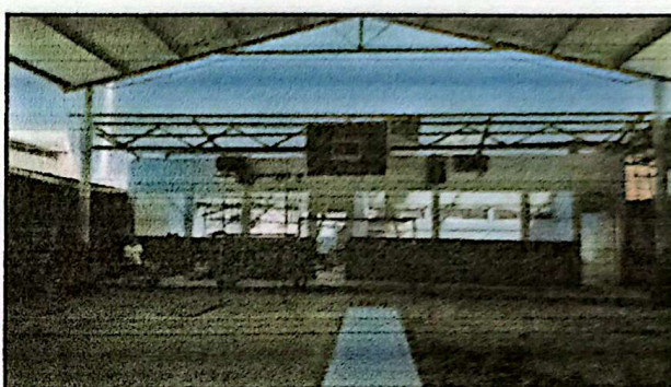
Foto 4. Sustitución de cubierta de lámina por lámina troquelada calibre 26. Lado Oeste sobre la 0 Avenida de la Zona 1: Aulas de Párvulos Etapa 6 B y 1o. C. Corredor e interior de las aulas en mención.
