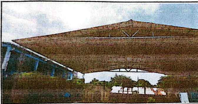
Foto #3: Sustitución de bases de madera por metal de tres metros. 10 bases
