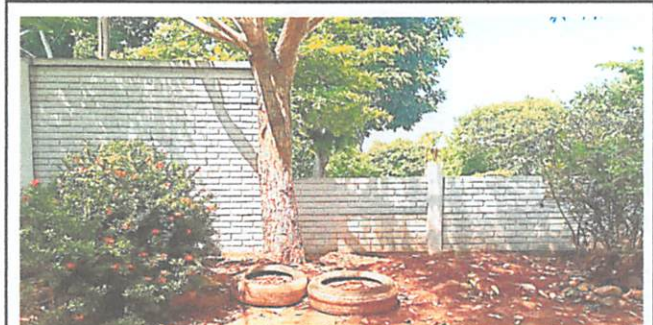
Foto 4: Sustitución de muro perimetral, placa manual de 2.00*0.50*0.05 m tipo ladrillo, poste barda de 3.15*0.15*0.15 m tipo H reforzado
