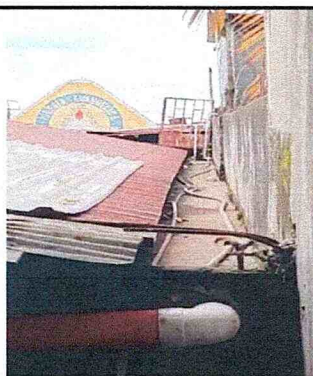
FOTO 3: IMPERMEABILIZACIÓN DE LOSA CON BLOQUEADOR DE AGUA AQUALOCK 10 AÑOS. 30 metros cuadrados.
