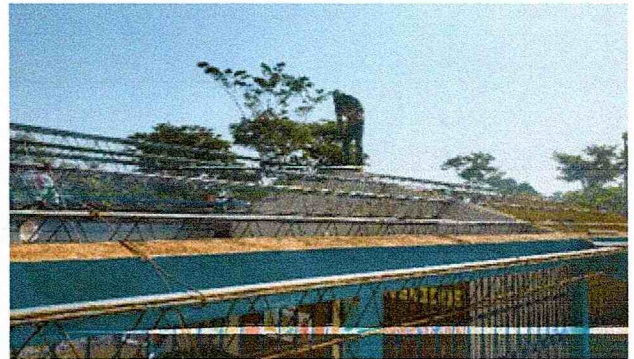
Foto 2: Sustitución de lámina, por lámina troquelada calibre 26.
