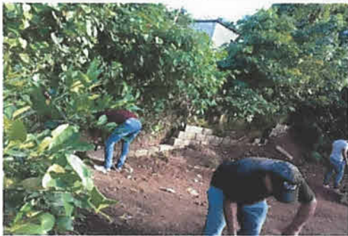
Reparación de muro de contención MC2-H=3.00 y losa de cimentación. 80M3 (Losa de cimentación: 27mx1.4mx1.25m=47.10m3 + Muro de Contención: 27mx2.6mx0.47m= 32.9m3)
