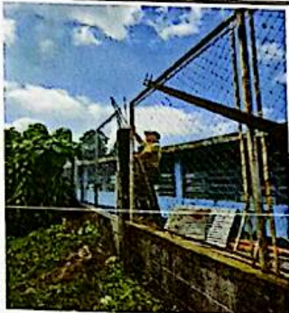
Foto1: Sustitución de reja perimetral de malla galvanizada de 2X2
