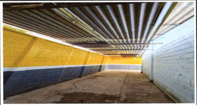
Foto 2: Sustrucción de cubierta de lámina troquelada de policarbonato calibre 26
