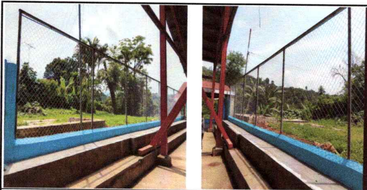
SUSTITUCION DE MURO PERIMETRAL CON TUBOS GALVANIZADOS DIAMETRO DE 2 PULGADAS MAS MALLA PERIMETRAL No. 2
