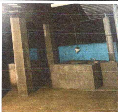
Sustitucion de losa concreto para rotoplas en base de rotoplas y piso de cocina
