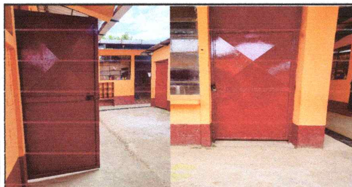
No.3 Reparación de puerta de metal Con tubo cuadrado de 1*1 + lámina 3/64
