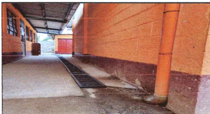
No.4 Reparación de cunetas de desfogue pluvial
