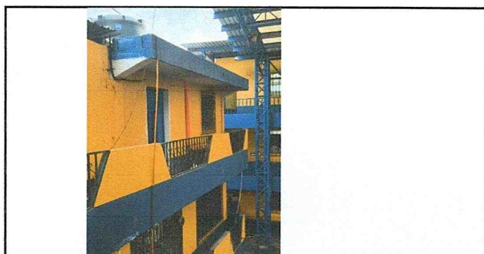
Instalación de bajante de drenaje de agua fluvial de losa.
