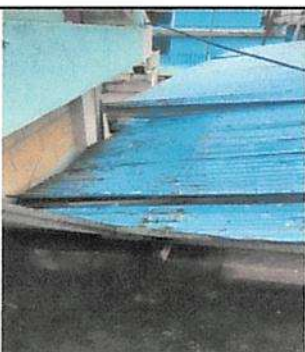
Sustitución de estructura de soporte de madera por metal tubo cuadrado de 3"x2"
