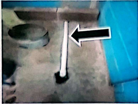
Foto 7: Instalación de 6 mts. de tubería PVC, Línea principal para migitorio 4" con recubrimiento de concreto en módulo 1
