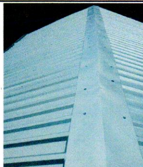
Foto 2: Sustitución de lámina por lámina troquelada calibre 26 sobre cocina
