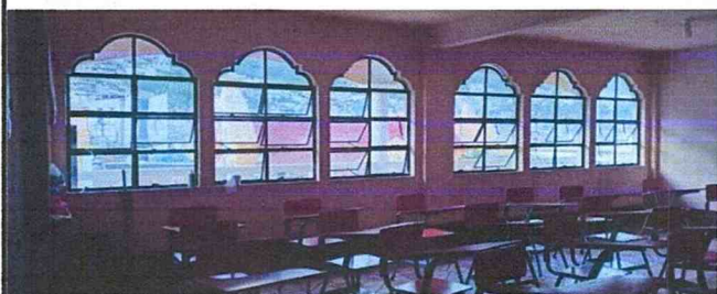
Sustitución de estructura de metal de ventana a pvc de 1.20 m2 cada ventana, tercer nivel
