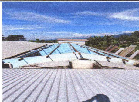
Foto 6: Sustitución de lamina troquelada en cubierta
