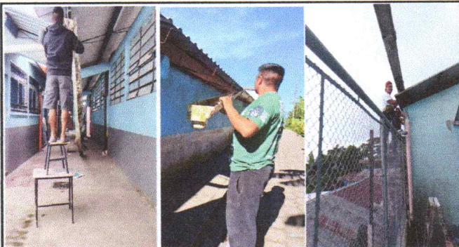
Foto1: Sustitución de de canal de metal en cubierta
