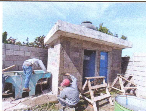
Mantenimiento de pared. Repello y acabados
