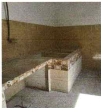
No.7 SUSTITUCIÓN DE PILA MOVIBLE POR PILA DE CONCRETO ARMADO CON RECUBRIMIENTO
