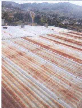
Sustitución de techo con lamina troquelada C26 recubierta de aluminio y zinc (incluye canaleta para bajada de agua)
