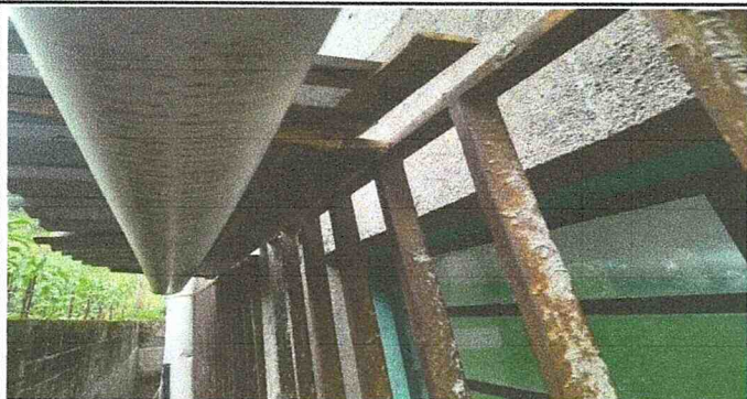
Sustitución de lámina acanalada y estructura de madera por estructura de metal y lámina troquelada en módulo 1
