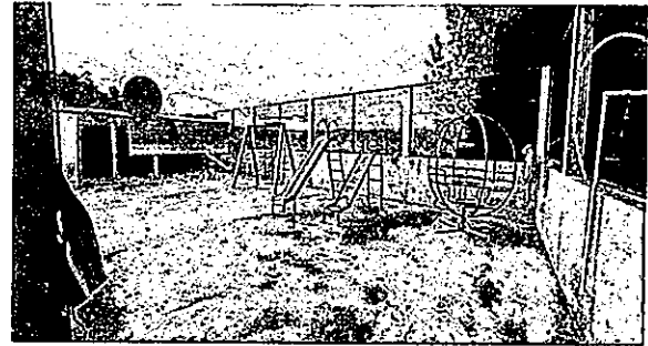
Mantenimiento correctivo en losa con concreto y aditivo para concreto viejo y nuevo con un 2 % de desnivel hacia aguas pluviales y acabado remolineado 168 m2. en patio tercer nivel - finalizado
