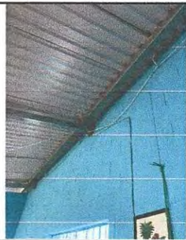
Reparación de cableado eléctrico CALIBRE 12 AWG sobre puesto en aulas módulo 1.
