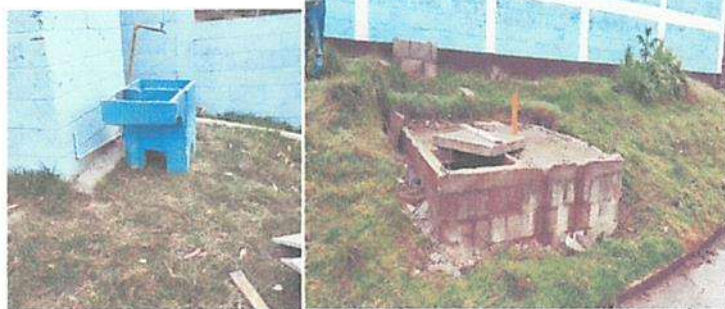
1.Sustitucion de pila de concreto 2. Aplicación y remozamiento de fosa septica ( repello, caja de cortina con block y tapadera, instalacion de tuberias de baños, cerndidos y tallados, revision de material de absorcion)
