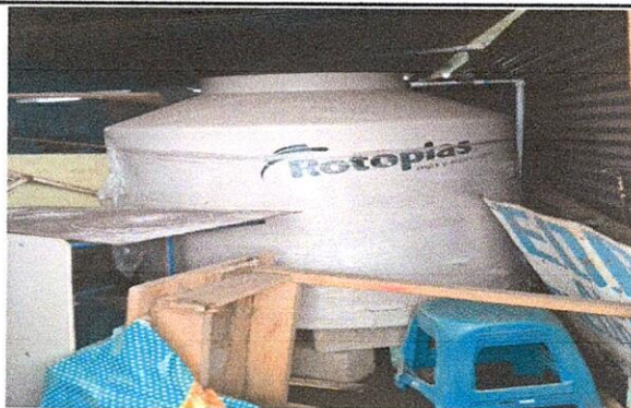
Sustitución de depósito de agua Rotoplas de 2,500 lts e instalación base de block
