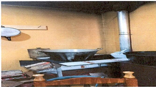
Sustitución de plancha ahorradora a plancha de 1.30 mts x 1.00 mts y 0.90 mts de alto, de concreto y ladrillo, con chimenea de tubo de concreto, en cocina del módulo 2
