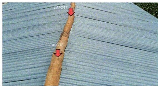
Sustitución de capote de lámina para lámina troquelada calibre 26 módulo A
