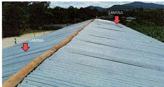
Sustitución de lámina, por lámina troquelada calibre 26 aulas módulo A
