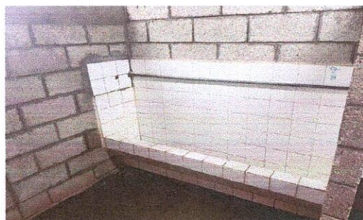
Sustitución de migitorio de concreto
