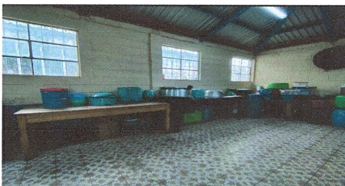
REMOZAMIENTO DE MESA DE CONCRETO CON DIMENSIONES (6.30X0.80X0.90)MT CON PUERTAS EN COCINA
