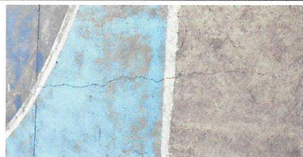
sustitución de piso de concreto T-0.10 mts 3000 psi
