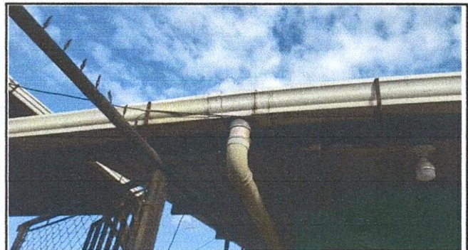
4. Sustitución de canal, por canal de PVC de alto caudal. Modulo 1 y 2. (30.5 m2).
