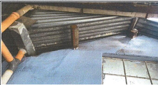
3. Sustitución de estructura portante, por estructura portante de costanera de 2" x 4" x 1.5mm. Modulo 3. (19.00 m2).
