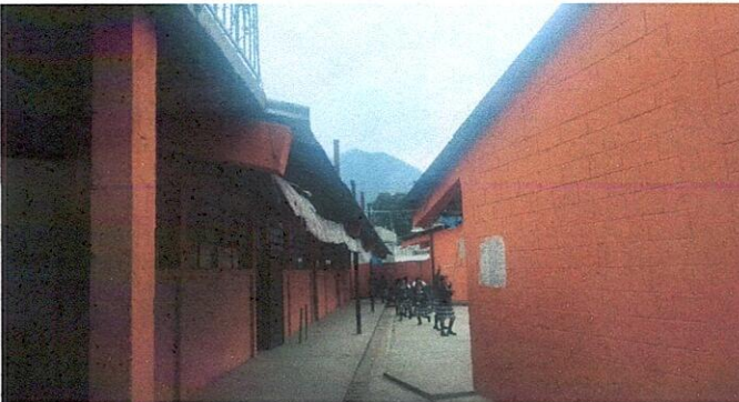
fabricación de 47mts de canales galvanizado calibre 26
