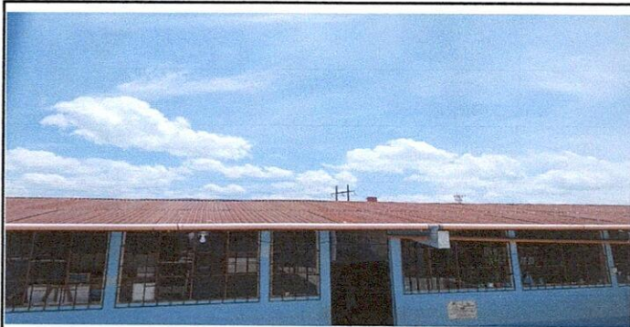
Foto 3: Sustitución de lamina, por lamina troquelada calibre 26 de módulo 3
