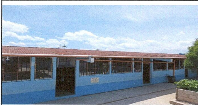
Foto 2: Sustitución de lámina, por lámina troquelada calibre 26 de módulo 3
