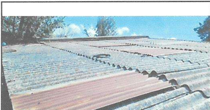
Sustitución de lámina existente por lámina troquelada calibre 26 de 1 metro de ancho útil por 98.20 mts de largo en Módulo 1
