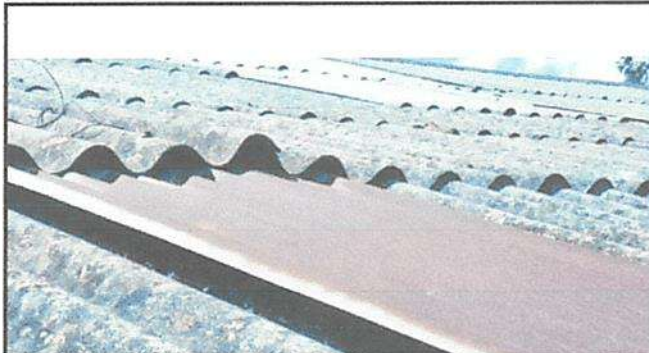
Sustitución de lámina existente por lámina troquelada calibre 26 de 1 metro de ancho útil por 98.20 mts de largo en Módulo 1
