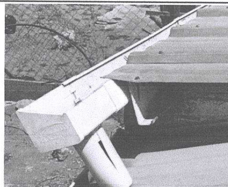
Sustitución de bajadas de agua de alto caudal con tubería de PVC de 3" y 4" en módulo de aulas 1.
