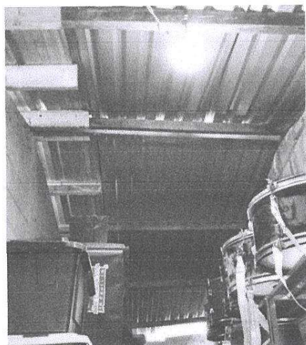
Sustitución de cielo falso de tablayeso en área de dirección; estructura de soporte de perfil omega y angular galvanizado, planchas de tablayeso de espesor de 1/2", cintas en uniones y pasta de yeso.
