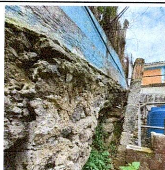
Desplazamiento del muro
