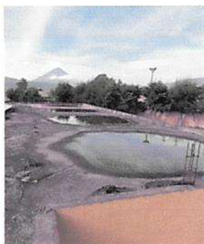
Impermeabilización de losa con Manto Asfáltico de 3mm con acabado de gravilla color terracota 10 años
