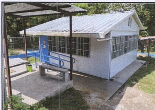
PISO MEJORAMIENTO DE TORTA DE CONCRETO
