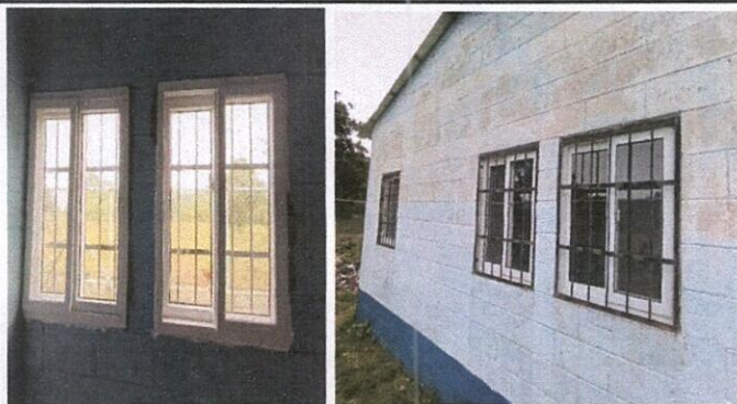
Foto 2: 2 tres vetanas de computación, medidas ancho 84.5 cm por 1.4 m de altura
