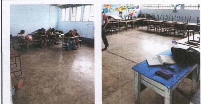
Foto 6: Aula 2 y 3 sustitución piso de cemento por piso cerámico, medidas del aula 2 5.88 por 9.97 y medidas del aula 3 7.27 por 7.22.
