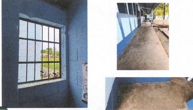
Foto 1: Una ventana de la dirección, medidas 84.5 por 1.4, pasillo grande 25.05 por 2.04, pasillo pequeño 2.63 por 1.03
