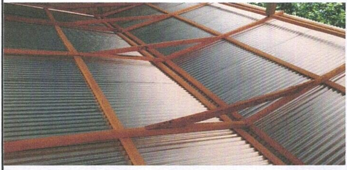
Foto: 2.2 Sustitución de estructura de soporte de madera, por metal
